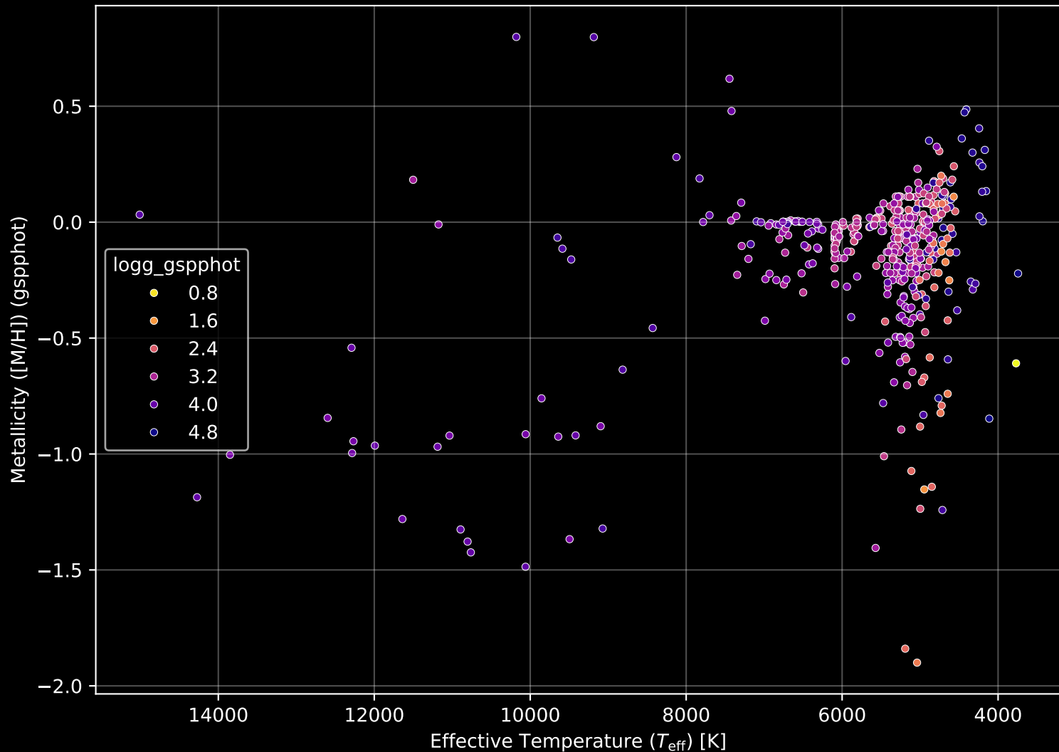
APOGEE DR17 Field: [210-04] Stellar Population Parameters (n= 452)
